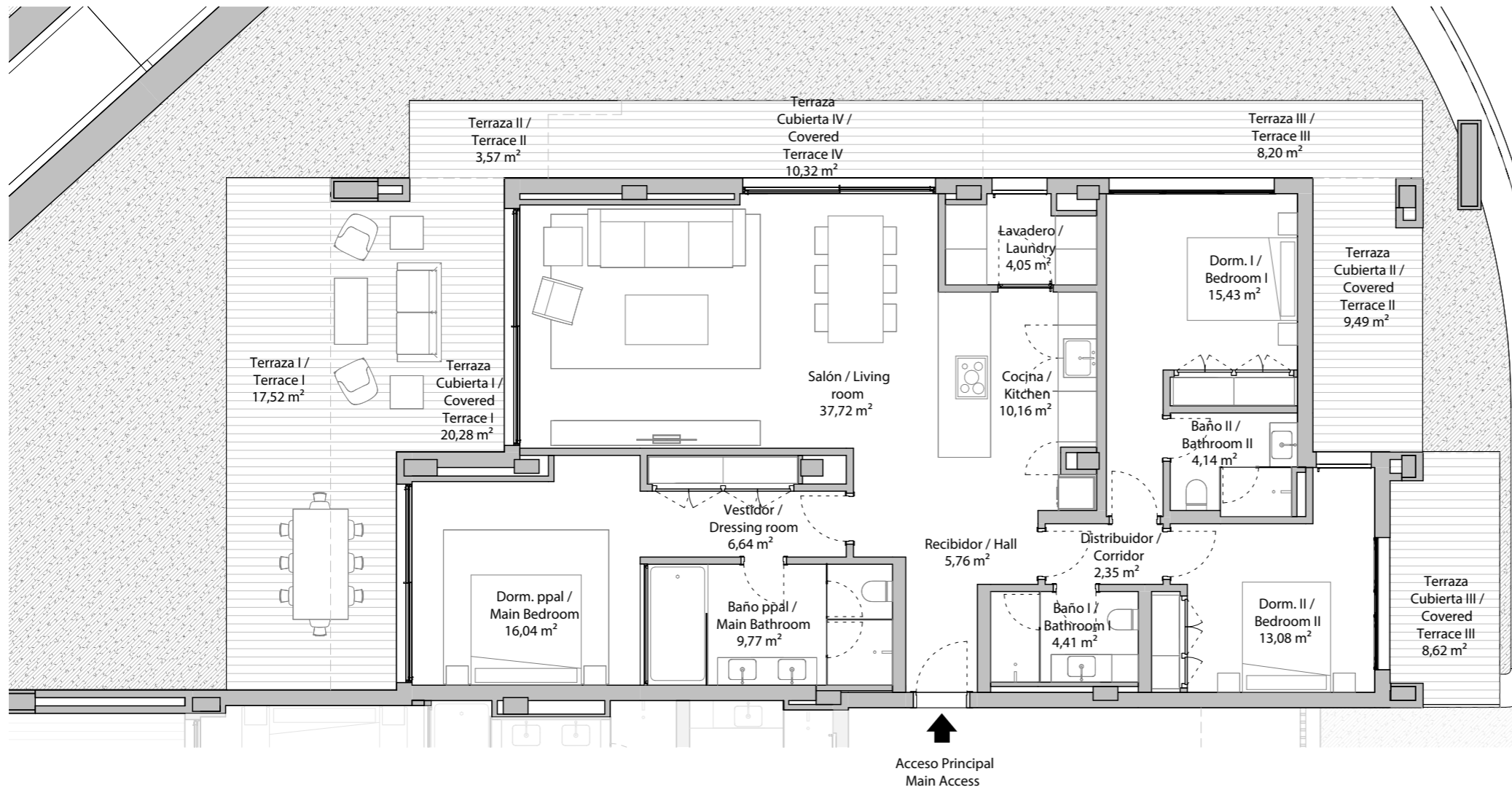
PLANTA VIVIENDA
